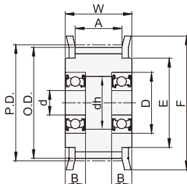
VTH01 双轴承
