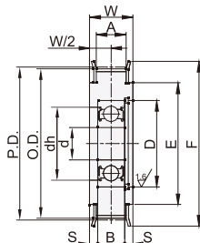
VTP01 单轴承
