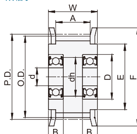
VTH01 双轴承
