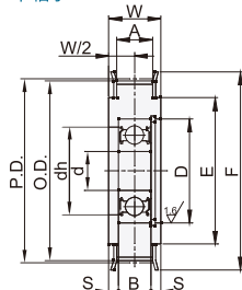
VTP01 单轴承
