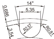
标准齿形
