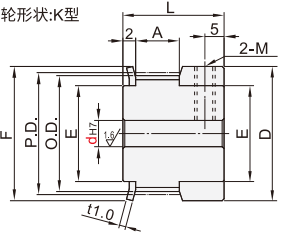
带轮形状:K型
