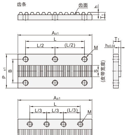
EAC01 (齿条+压板)
