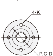
螺孔型 AJP85/86
