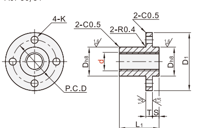
嵌入型 AJP80/81
