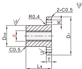
螺孔型 AJP85/86
