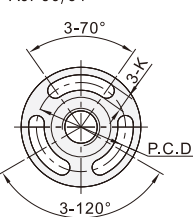
腰孔型 AJP90/91
