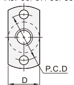
双孔对边型 AJP66/67/68/69
