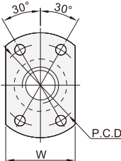
四孔对边型
