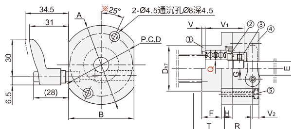
防转动固定件 AHF08
