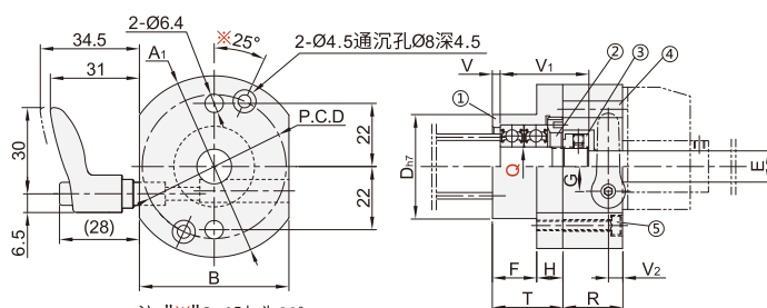
AHF10 大型位置显示器安装用防转动固定件
