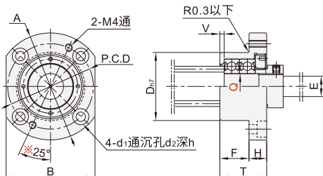
支座组件主体 AHF03
