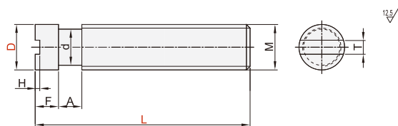
一字槽带环槽全牙型 AFH01/11
