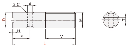
带一字槽半牙型 AFC01/11
