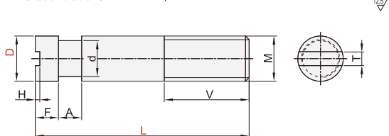
一字槽带环槽半牙型 AFG01/11
