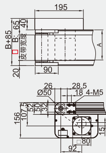
■ 调速\定速\变频电机尺寸(参考值)
