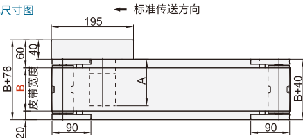
■ 整机尺寸图
