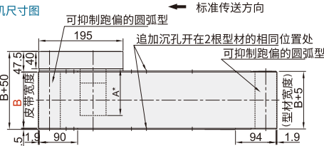
■ 整机尺寸图
