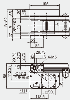
■ 调速\定速\变频电机尺寸(参考值)
