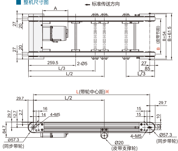
■ 整机尺寸图
