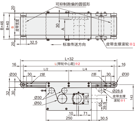
■ 整机尺寸图
