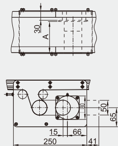
■ 步进电机尺寸(单位:mm)
