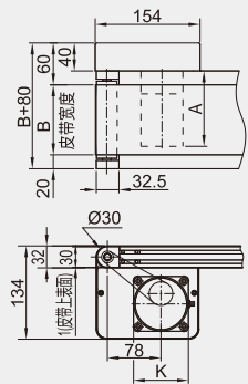
■ 步进电机尺寸(单位:mm)
