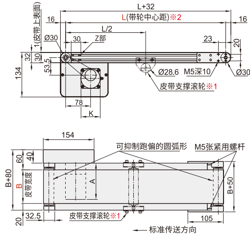
■ 整机尺寸图
