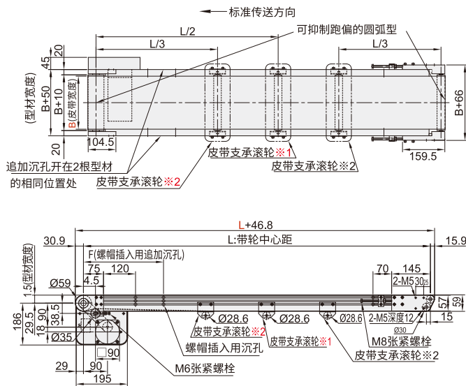
■整机尺寸图
