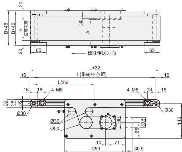
■ 整机尺寸图
