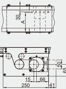
■ 调速\定速\变频电机尺寸(参考值)
