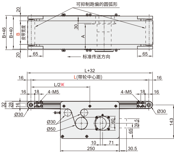
■ 整机尺寸图
