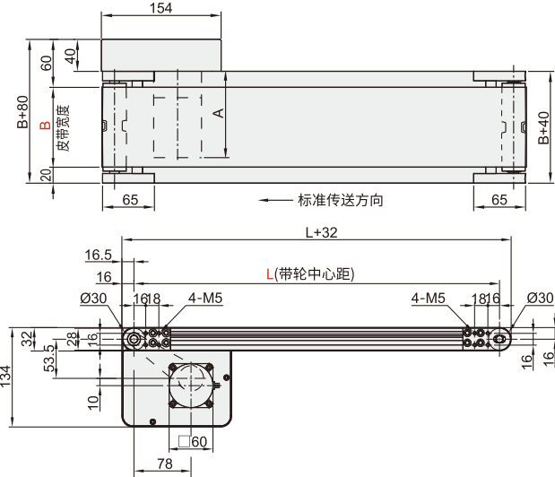
■ 整机尺寸
