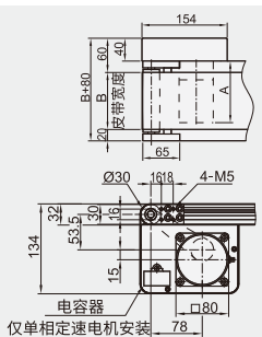
■ 调速\定速\变频电机尺寸(参考值)
