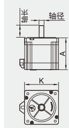
■ 步进电机尺寸(单位:mm)
