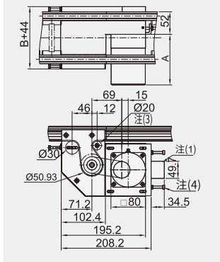
■ 步进电机尺寸(单位:mm)
