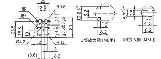
■ 双槽型材截面放大
