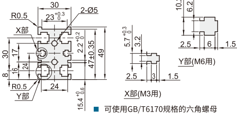
■ 三槽型材截面放大
