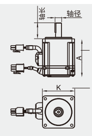
■ 伺服电机尺寸(参考值)
