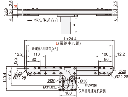
■ 三槽整机尺寸图
