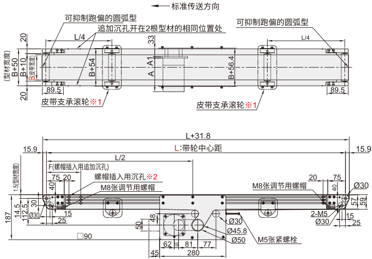
■ 整机尺寸图
