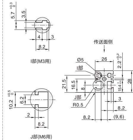
■ 型材截面放大图
