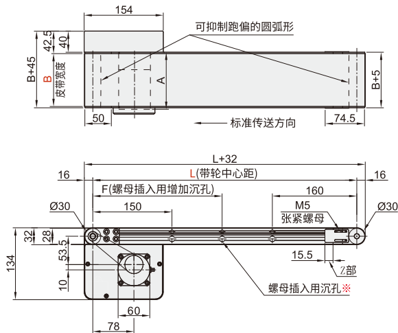
■ 整机尺寸图
