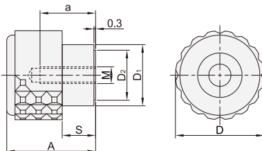
带台阶 内螺纹型 SJK33
