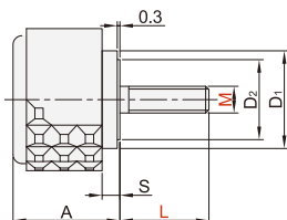
无台阶 外螺纹型 SJK21/22
