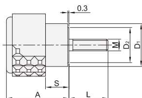
带台阶 外螺纹型 SJK31/32
