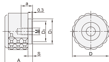
无台阶 内螺纹型 SJK23
