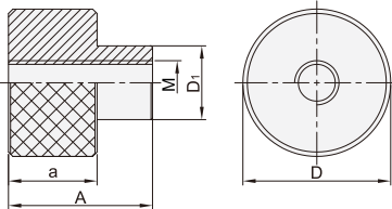
带台阶 内螺纹型 SJK12
