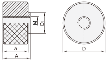
无台阶 内螺纹型 SJK02
