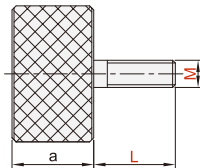
无台阶 外螺纹型 SJK01
