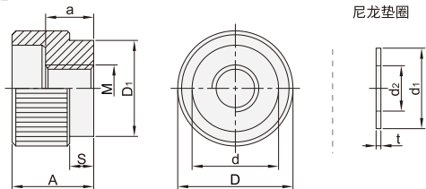
尼龙垫圈
