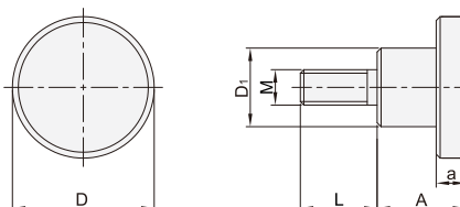
外螺纹型 带台阶 SJG11
