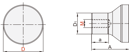
内螺纹型 无台阶 SJG01
