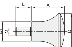
外螺纹型 CSJA32
