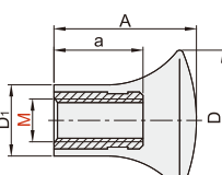
内螺纹型 SJA33
