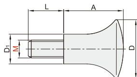
外螺纹型 CSJA31
