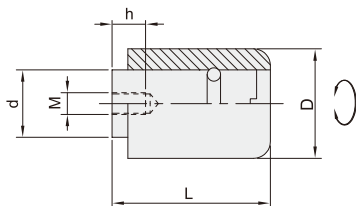
内螺纹型 SSH01
