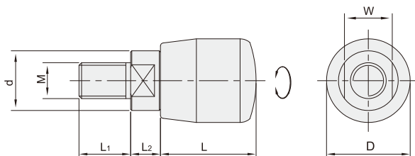
外螺纹带扳手槽型 SSH11
