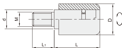
外螺纹型 SSH02
