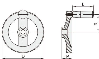
D=140~200
