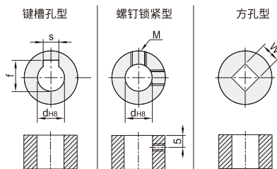
键槽孔型
