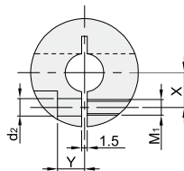
夹紧位置详细尺寸
