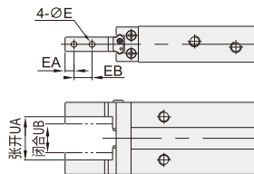
通孔安装型(N型) Φ6
