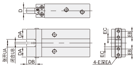
底部安装型(F型) Φ6
