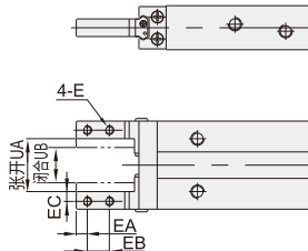
侧面安装型(B型) Φ6
