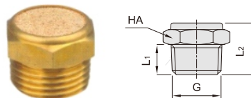
HDCG11-SLM-G微型消声器
