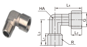
HDCF71-BLM 内外螺纹弯头
