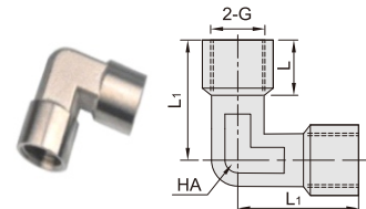
HDCF72-BLF 双内螺纹直角弯头
