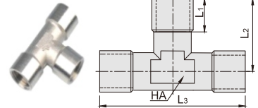
HDCF51-BF 内螺纹三通
