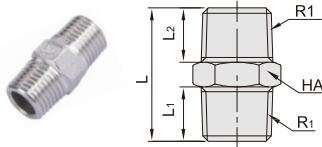
HDCF11-BB 双外螺纹直通
