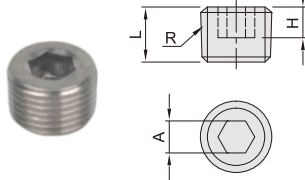
HDCF41-BP 内六角堵头
