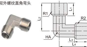
HDCF73-BL 双外螺纹直角弯头
