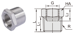
HDCF31-BD 内外螺纹直通
