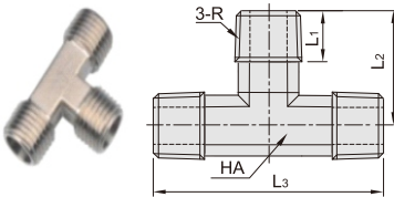
HDCF61-BT 内外螺纹三通
