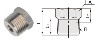
HDCF21-BZ 外六角堵头
