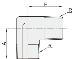
外螺纹等径 HDCP51
