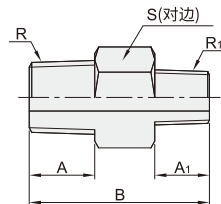
外螺纹等径 HDCP51
