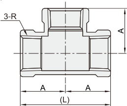
T型接头 内螺纹 HDCX11
