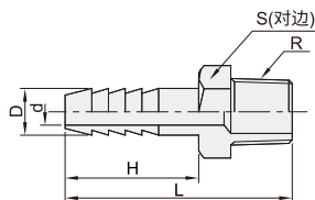
直接头 外螺纹 HDCX01
