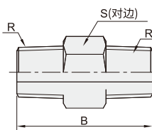
外螺纹异型 HDCP01
