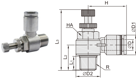
HDCC71-SSD不锈钢节流阀
