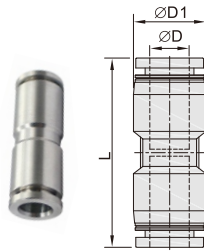
HDCC51-SSU联管直通
