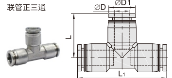
HDCC31-SSE 联管正三通
