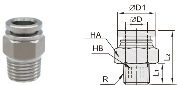
HDCC01-SSC 螺纹直通
