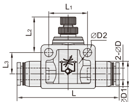
HDCB31-CSU管道阀
