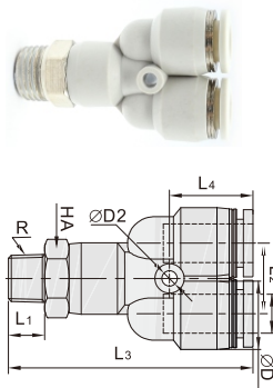
HDCA61-CPX Y型螺纹三通
