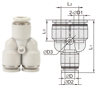
HDCA72-CPY 塑料Y三通
