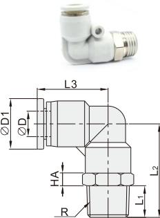
HDCA21-CPL L型螺纹弯头
