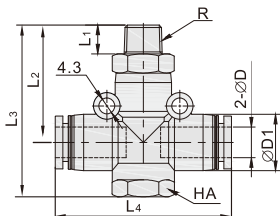
HDCA41-CPGT外六角双向接头
