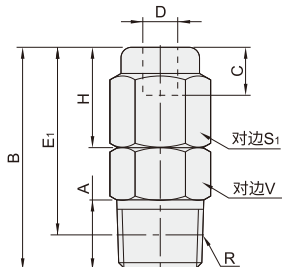
直接头/外螺纹 HDCY01
