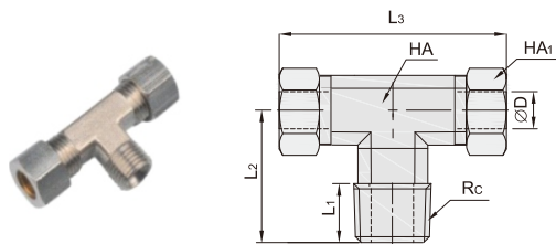
HDCE27-CKT 卡套螺纹正三通
