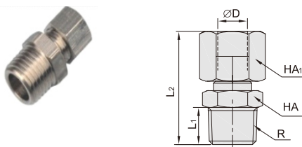
HDCE25-CKC 卡套螺纹直通
