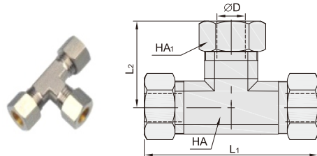
HDCE28-CKE 卡套三通
