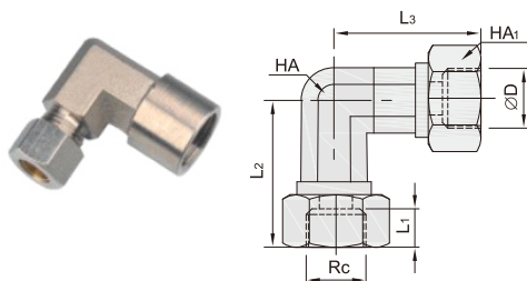
HDCE26-CKLF 卡套内螺纹弯头
