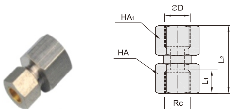
HDCE22-CKF 卡套螺纹直通
