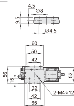
A-A视图
