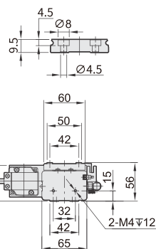
A-A视图
