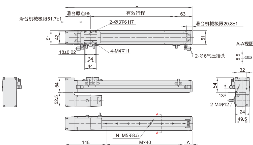
BM马达下折
