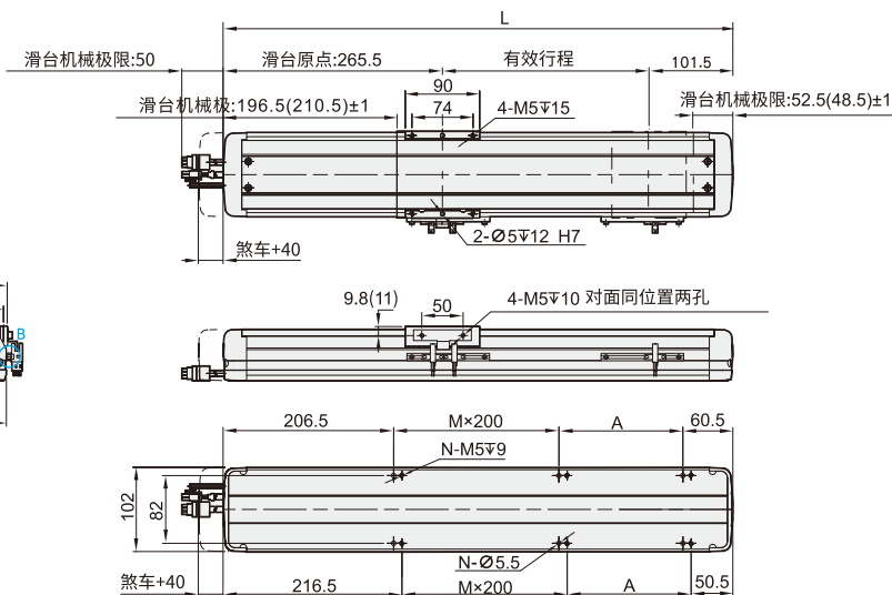
B视图
