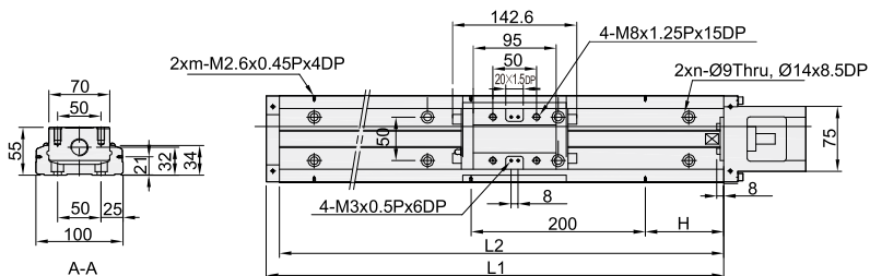
■ 不含护盖尺寸图
