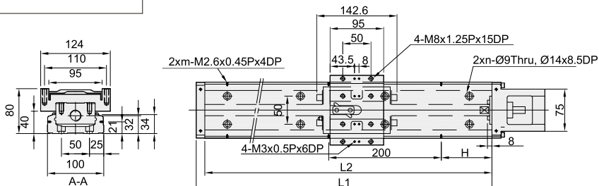
■ 含护盖尺寸图
