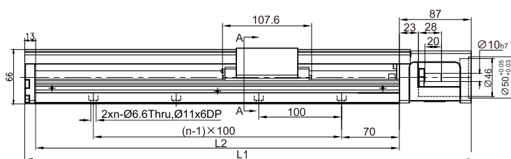
■ 不含护盖尺寸图
