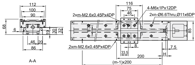
■ 含护盖尺寸图
