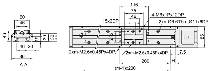
■ 不含护盖尺寸图
