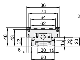
■ 含护盖尺寸图
