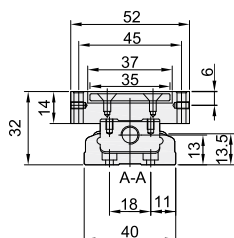
■ 含护盖尺寸图
